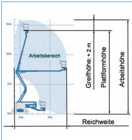
Bild 4-3: Arbeitshöhe
