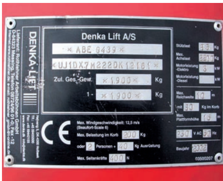
Bild 4-1: Fabrikschild
