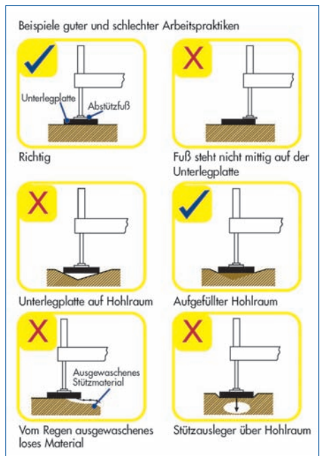
Bild 4-5: Beispiele zur Abstützung
